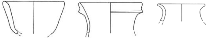
Fig. 20. Vasetti miniaturistici. A sinistra coppetta in ceramica a vernice rossa; al centro piccolo craterisco in ceramica a vernice nera; a destra olpetta in ceramica depurata (scala 1:2).
