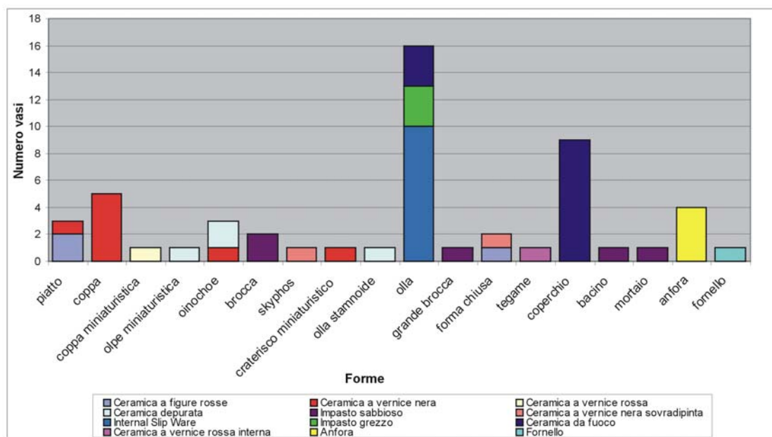
Fig. 1. Diagramma relativo alle forme funzionali attestate, per le quali viene indicato il numero dei vasi ad esse riferibili. I diversi colori delle colonne rappresentano le classi ceramiche in cui sono realizzate le forme.
