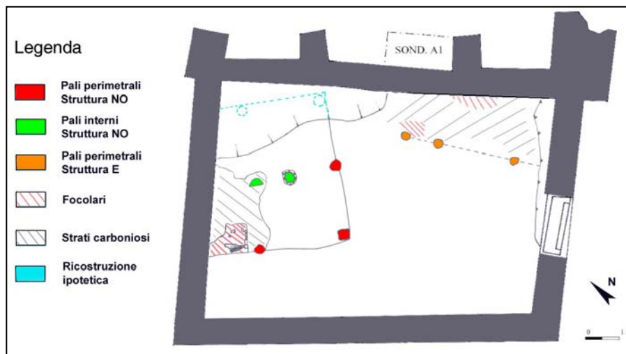
Fig. 10. Settore A, edificio I. planimetria delle evidenze relative alle strutture in legno (elaborazione grafica M. Battisti)
