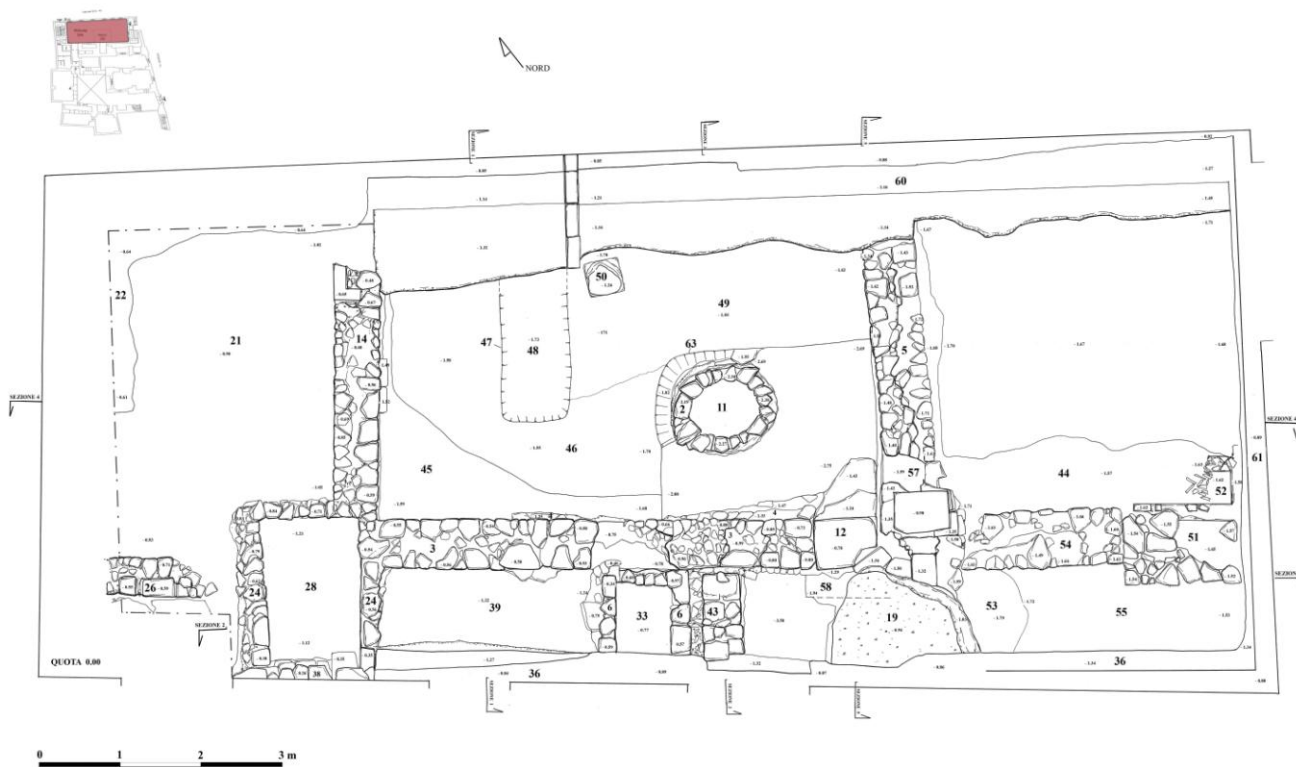
Fig. 8. Planimetria generale delle strutture rinvenute nel corso delle indagini svolte negli anni 2009 e 2010.
