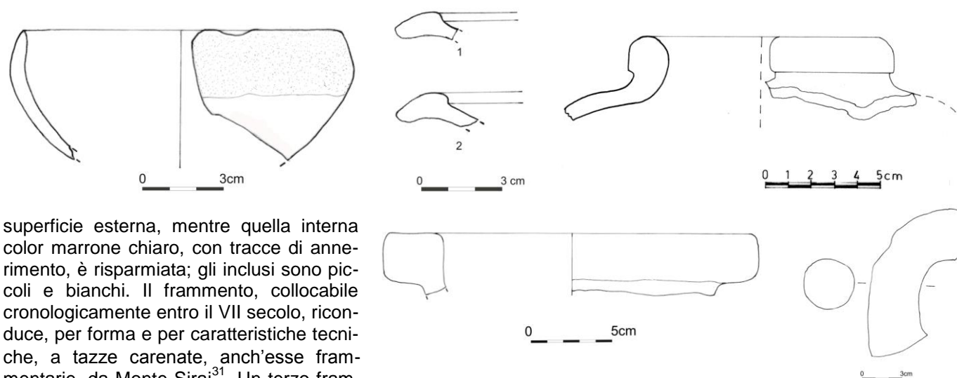
Figg. 11-15. Coppa a profilo curvilineo, piatti, anfora fenicia, anfore corinzie da Posada.
