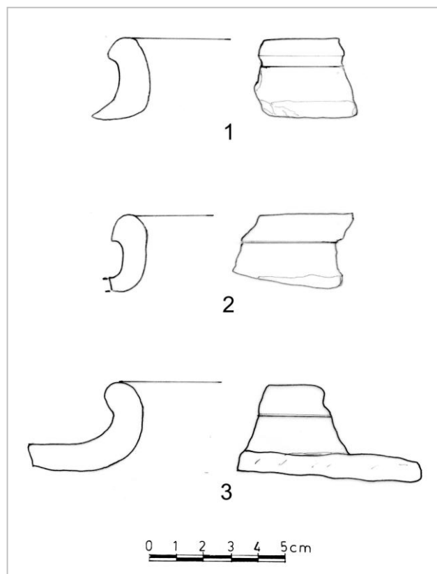
Fig. 4. Orli d'anfora tipo Sant'Imbenia da Posada.
