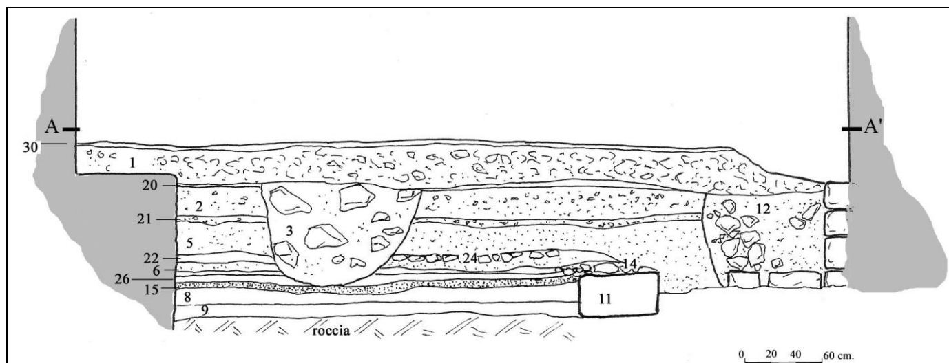
Fig. 3. Lecce, via delle Giravolte. Sezione dello scavo.
