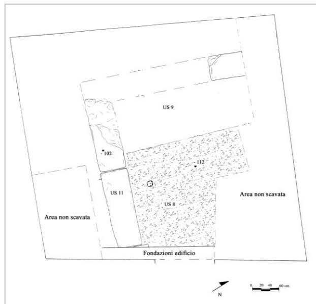
Fig. 4. Lecce, via delle Giravolte. Pianta dello scavo (Periodo 1).
